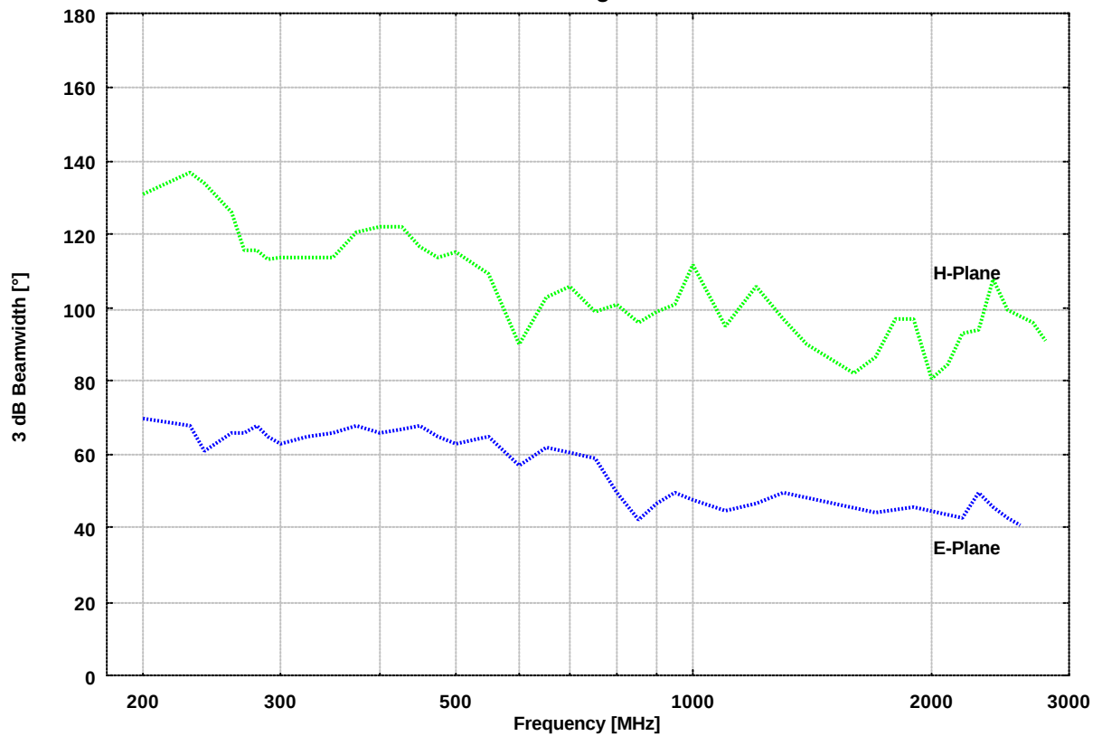
3 dB Öffnungswinkel:
